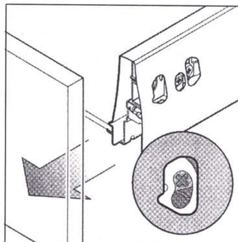
Afmonter front
