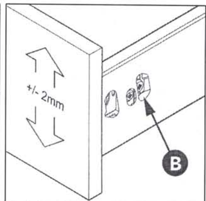
Højdejustering
