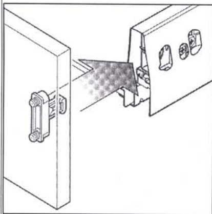
Montering af front
